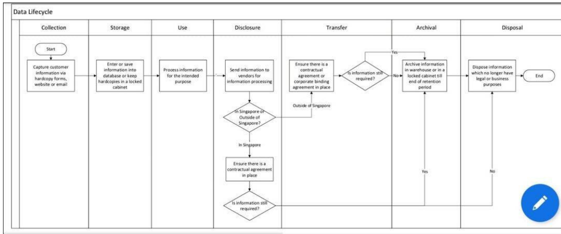
รูปที่ 1 ตัวอย่าง Data Flow ตาม Data Lifecycle
